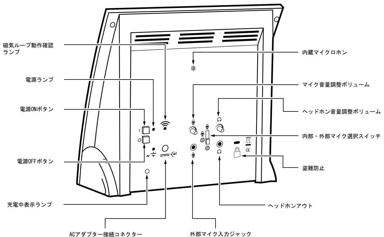
PLA 90 背面
